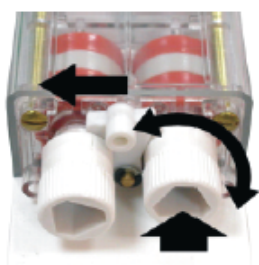
3- Desplazar separador lateralmente, subir regulador derecho y girar hasta el final de carrera ideal. Una vez fijado el final de carrera, bajar el regulador
