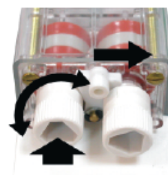
2- Comprobar que las rulinas están alineadas en posición 0
