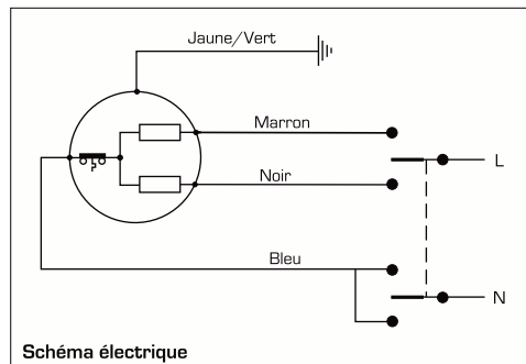
Schéma électrique
